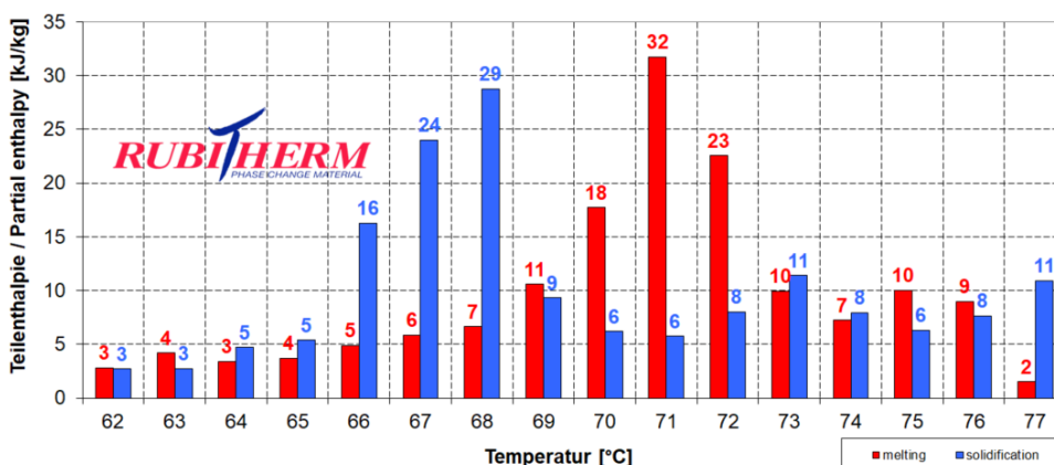
Beispiel / example: SP70 Teilenthalpie / Partial enthalpy distribution*
