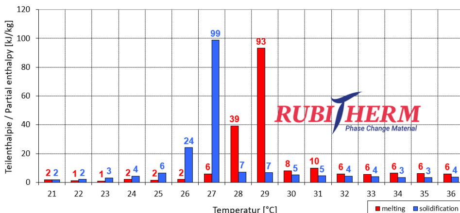
Beispiel / example: SP29Eu Teilenthalpie / Partial enthalpy distribution*
