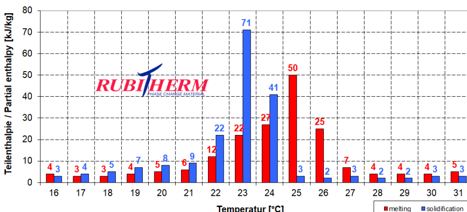
Beispiel / example: SP25E2 Teilenthalpie / Partial enthalpy distribution*
