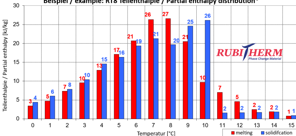
Beispiel / example: RT8 Teilenthalpie / Partial enthalpy distribution*
