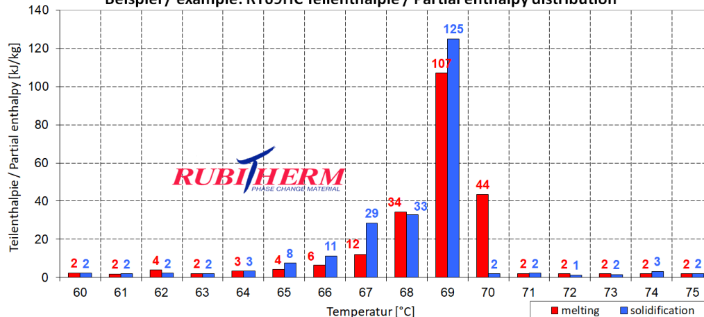
Beispiel / example: RT69HC Teilenthalpie / Partial enthalpy distribution*
