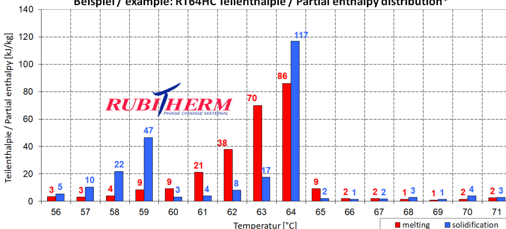
Beispiel / example: RT64HC Teilenthalpie / Partial enthalpy distribution*
