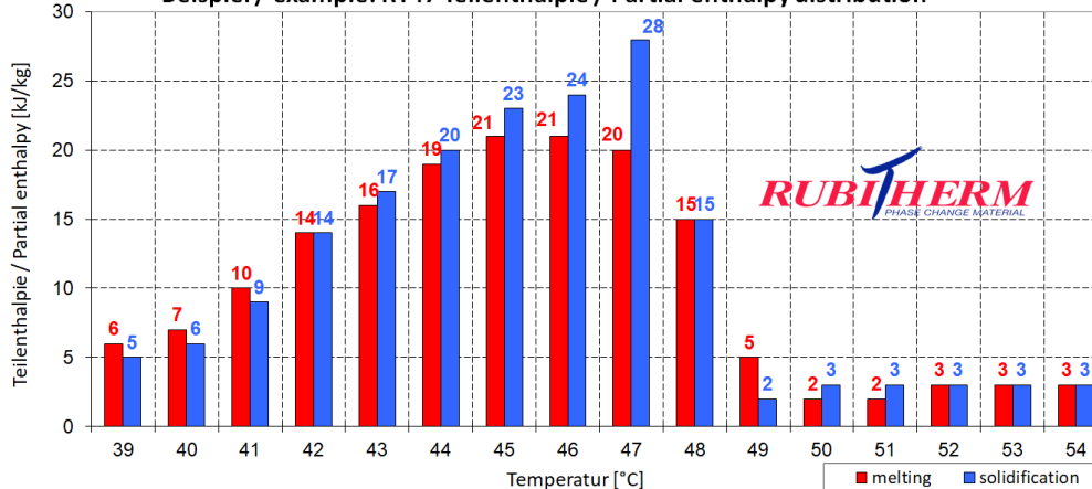
Beispiel / example: RT47 Teilenthalpie / Partial enthalpy distribution
