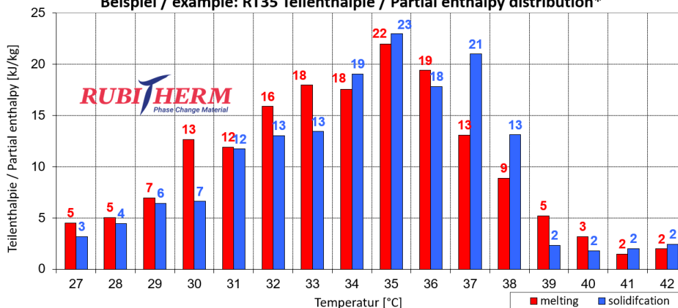
Beispiel / example: RT35 Teilenthalpie / Partial enthalpy distribution*
