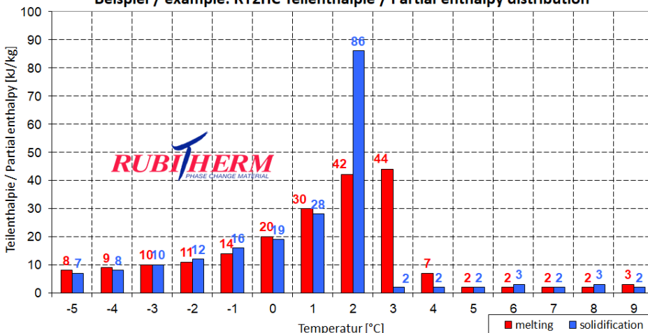
Beispiel / example: RT2HC Teilenthalpie / Partial enthalpy distribution
