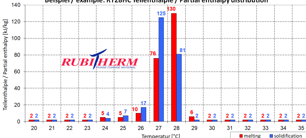
Beispiel / example: RT28HC Teilenthalpie / Partial enthalpy distribution
