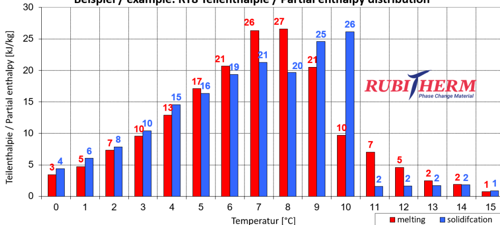
Beispiel / example: RT8 Teilenthalpie / Partial enthalpy distribution*
